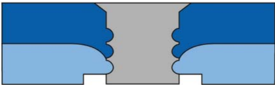
383_018 Kerb-Konus Nietverbindung
