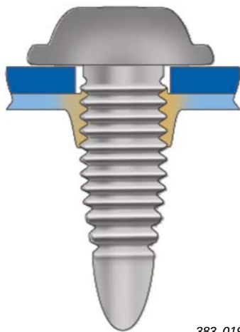
383_019 Flow-Drill Schraubverbindung
