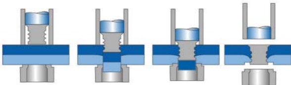
Prozessablauf Vollstanznieten
