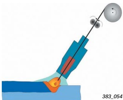
Prozessablauf MIG-Schweißen
