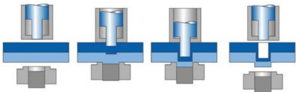
Prozessablauf Clinchen
