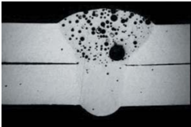
Schliffbild einer Laserschweißnaht mit Laser Clean (oben) und ohne Reinigung (unten)
