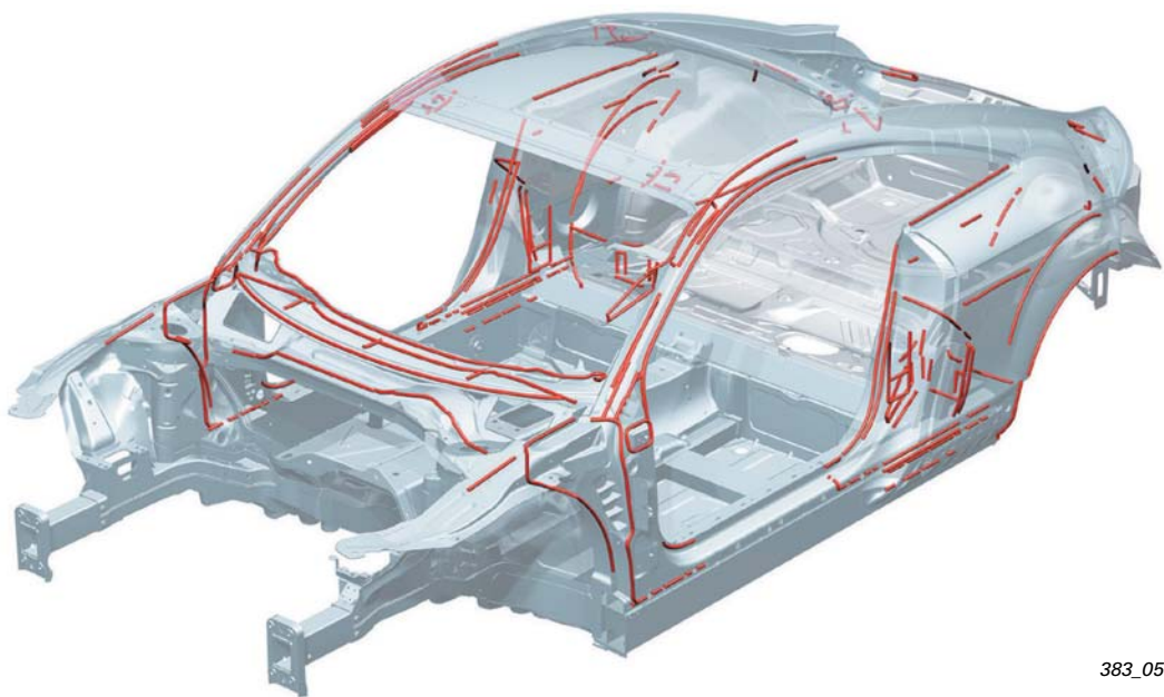
Einsatzbereiche Strukturkleber
