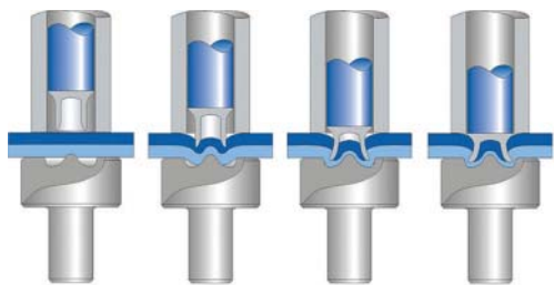
Prozessablauf Stanznieten
